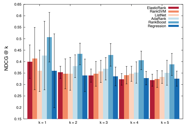
(b) TD2004
